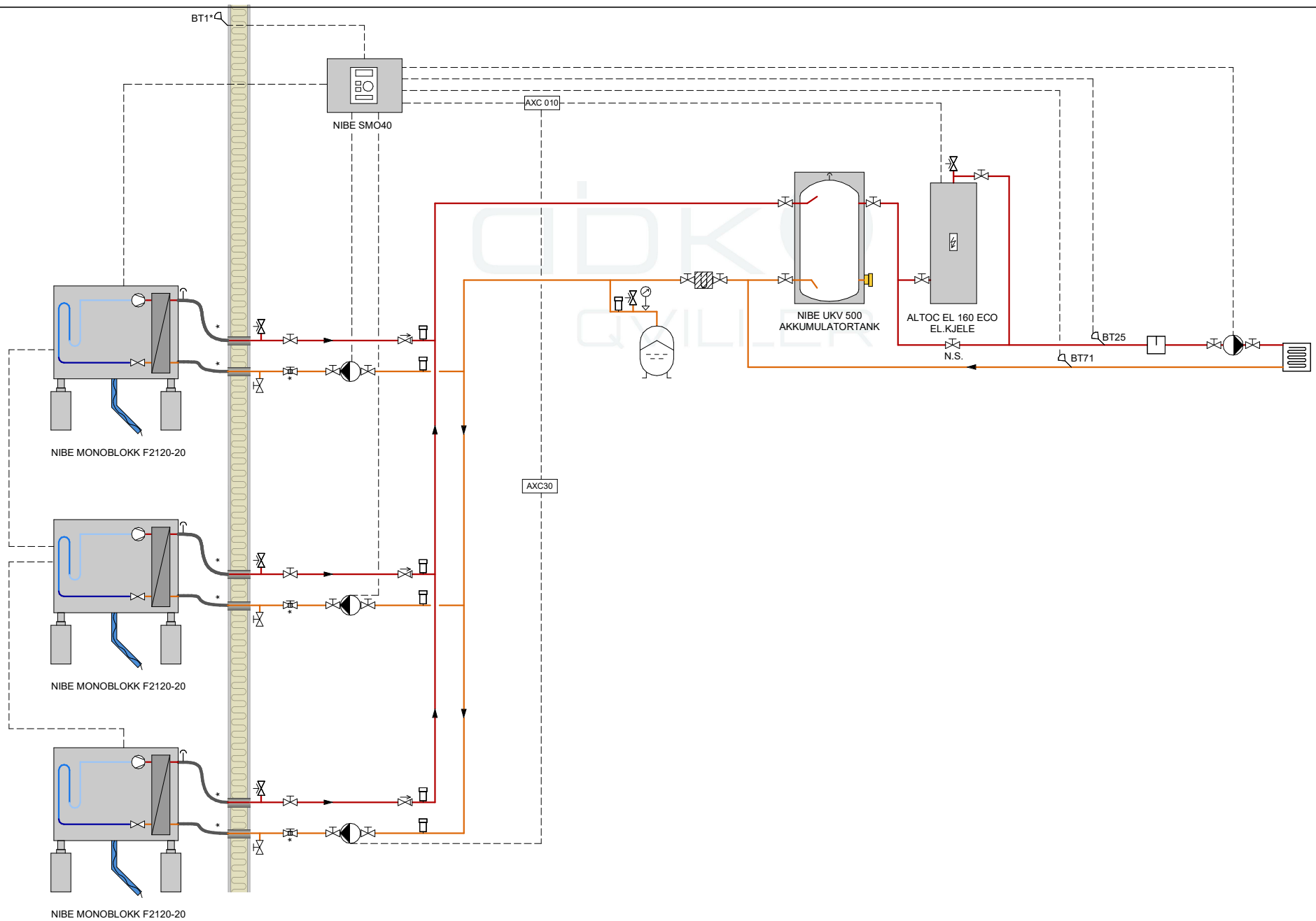
NIBE MONOBLOKK F2120-20
